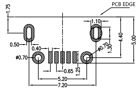
PCB图仅供参考
