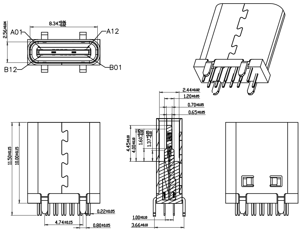
截面 1-1
