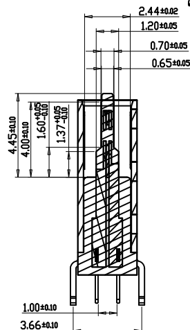
截面 1-1
