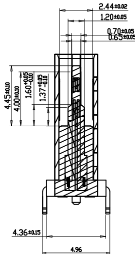
截面 1-1
