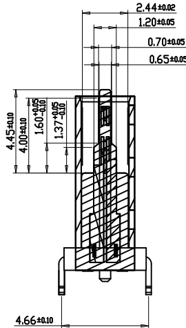
截面 1-1
