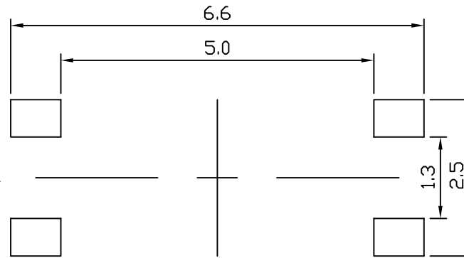
P.C.B LAYOUT
