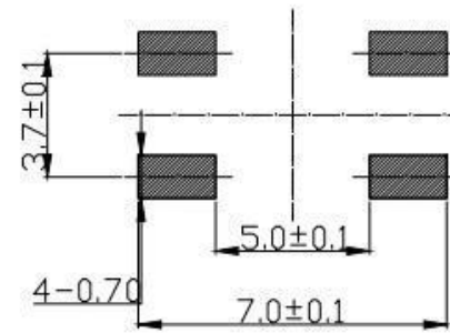
P.C.B 板焊接图
