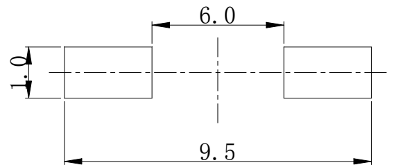
P.C.B 板焊接图
